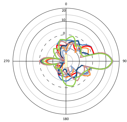
V-pol Elevation
